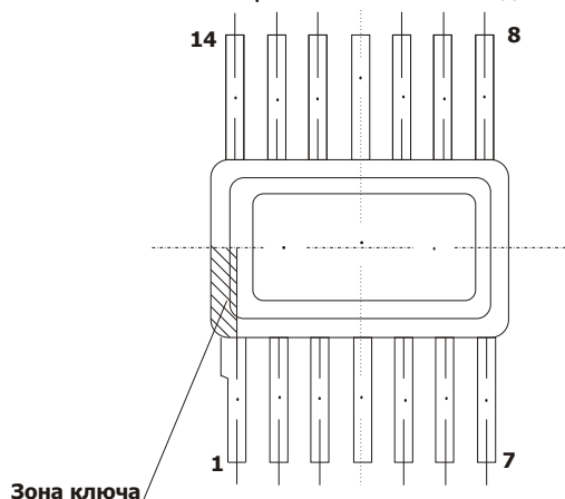
Схема расположения выводов
