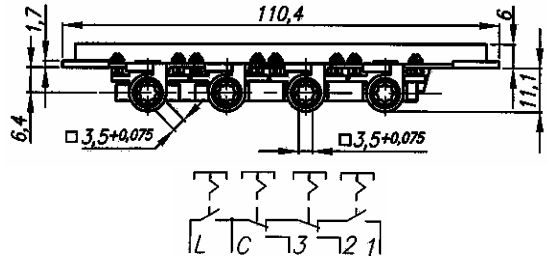
Габаритные размеры, электрическая схема коммутации
