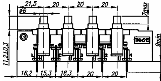
Габаритные размеры, электрическая схема коммутации
