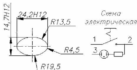
Разметка для крепления, схема коммутации
