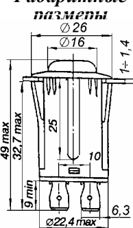
Габаритные размеры
