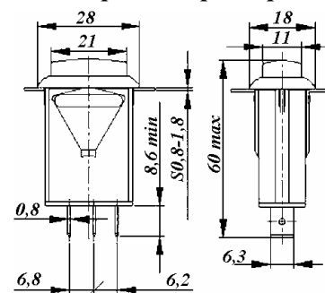
Габаритные размеры
