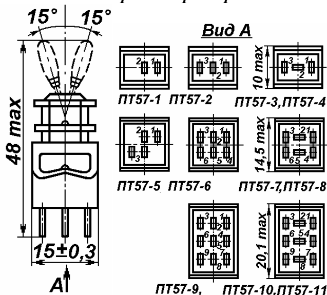
Габаритные размеры
