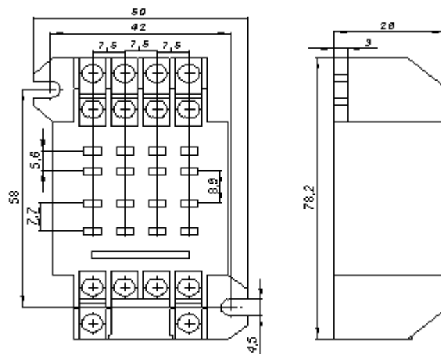
Габаритные размеры
