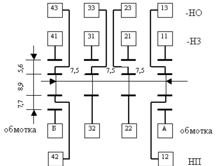
Схема соединений и шаг выводов реле РЭК59
