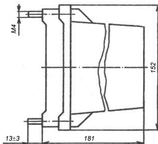
Переднее присоединение
