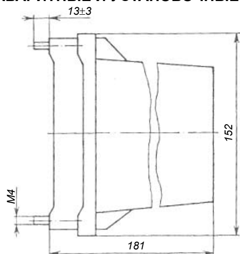
Заднее присоединение
