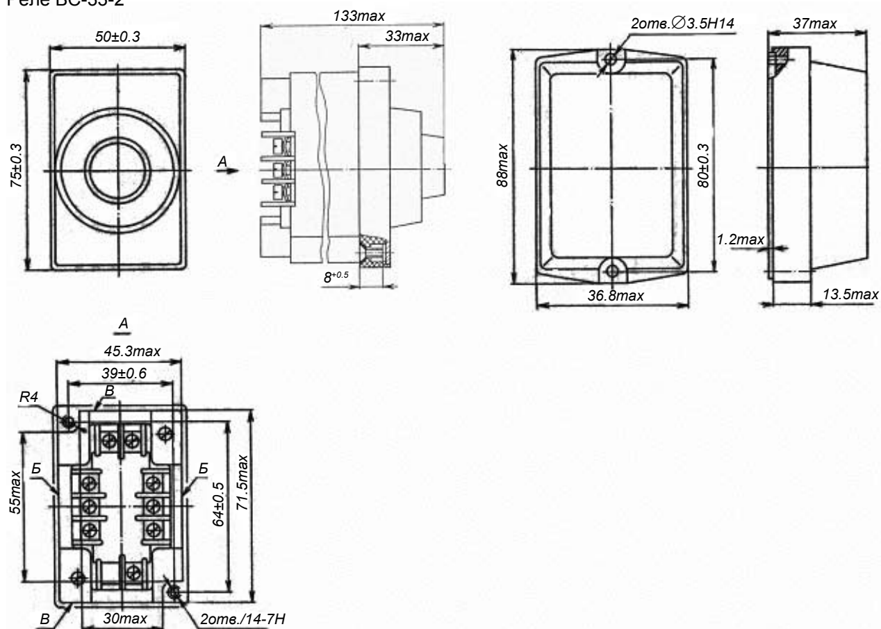
Реле ВС-33-2
