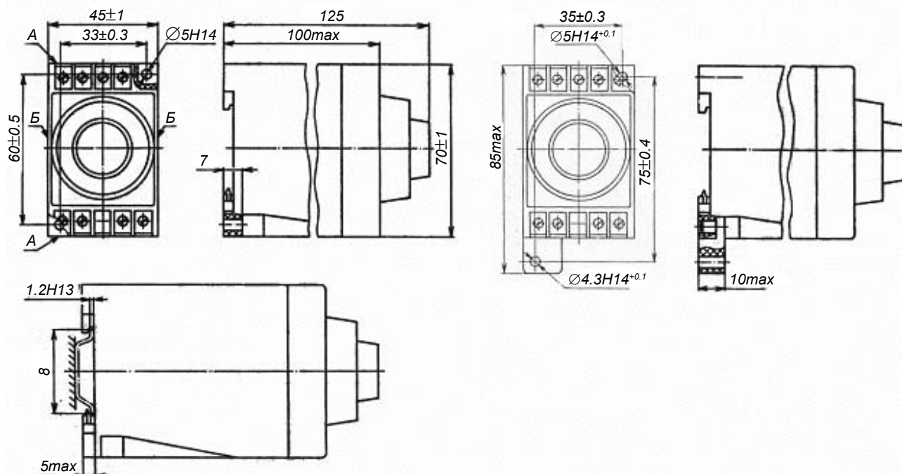
Реле ВС-33-1
