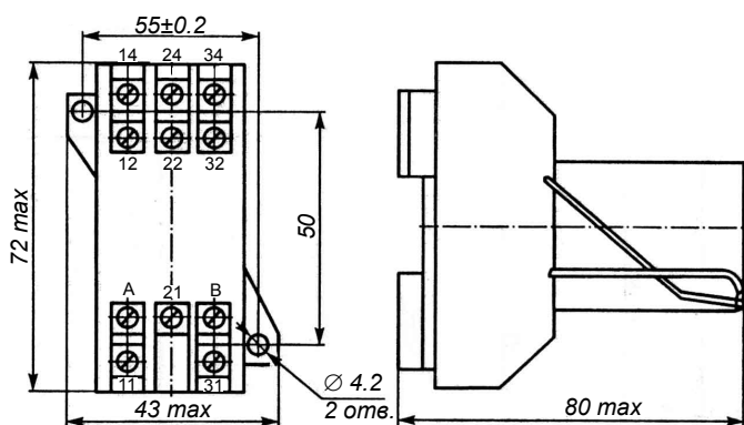
Реле с 3-мя переключающими контактами с розеткой тип 2
