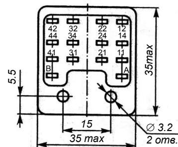
Реле с 4-мя переключающими контактами с розеткой тип 1
