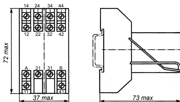
Реле с 4-мя переключающими контактами с розеткой тип 2
