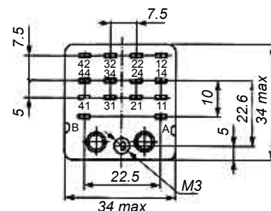
Реле с 4-мя переключающими контактами
