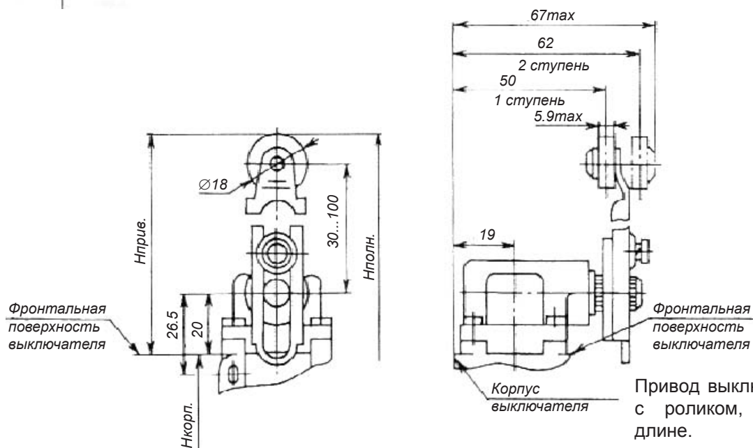
Привод выключателя типа рычаг, регулируемый по длине. Высота привода H_{прив.} \leq 170\text{мм} .
