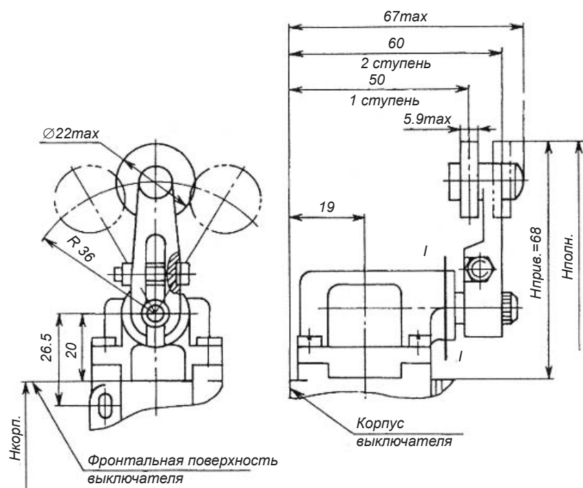
Привод выключателя типа рычаг с роликом. Высота привода H_{прив.} = 68\text{мм} .
