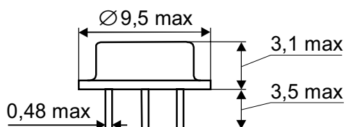
Корпус ТО-39
