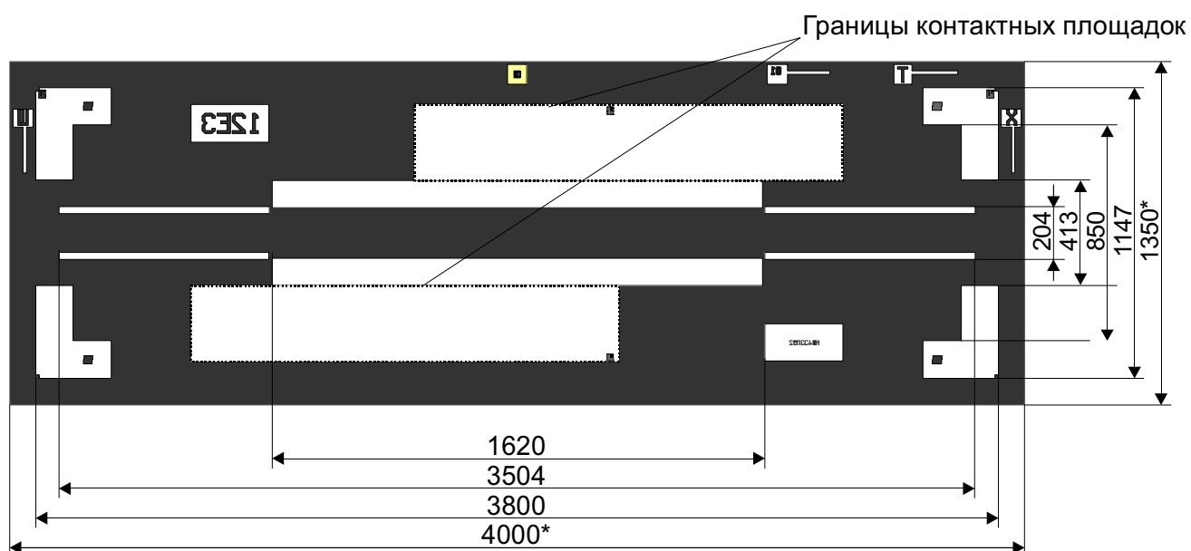
Чертеж кристалла на пластине
