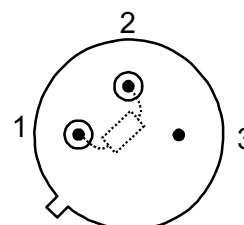
Цоколевка
