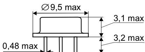
Корпус ТО-39
