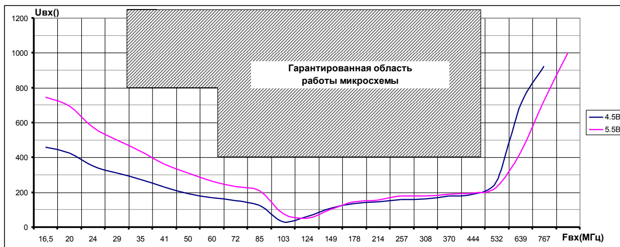
Рис. 9. Типовая зависимость минимального входного напряжения от частоты сигнала и область гарантированной работы ИС по входу Fin.
