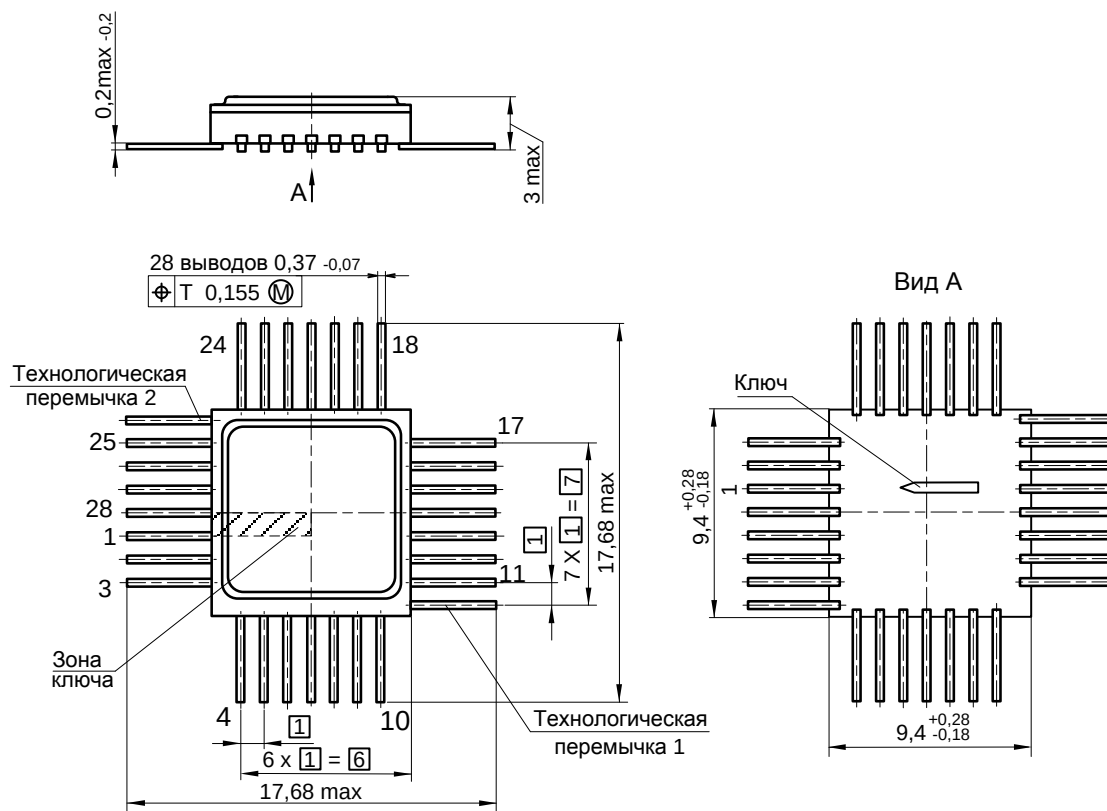
Рис. 10. Корпус H09.28-1В
