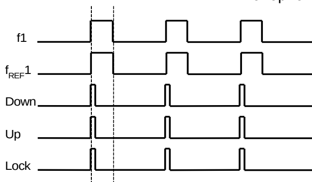
Рисунок 4. Сигналы ведомого и опорного генераторов совпадают
