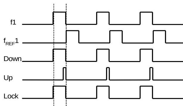
Рисунок 2. Сигналы ведомого генератора отстают от сигналов опорного генератора
