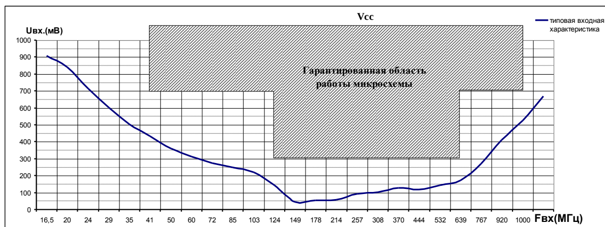
Рис. 7. Типовая зависимость минимального входного напряжения от частоты сигнала и область гарантированной работы ИС по входу Fin .
