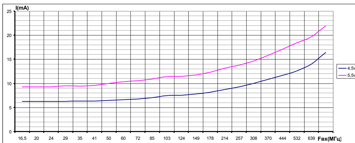
Рис. 8. Типовая зависимость тока потребления от входной частоты при напряжении питания 4,5В и 5,5В
