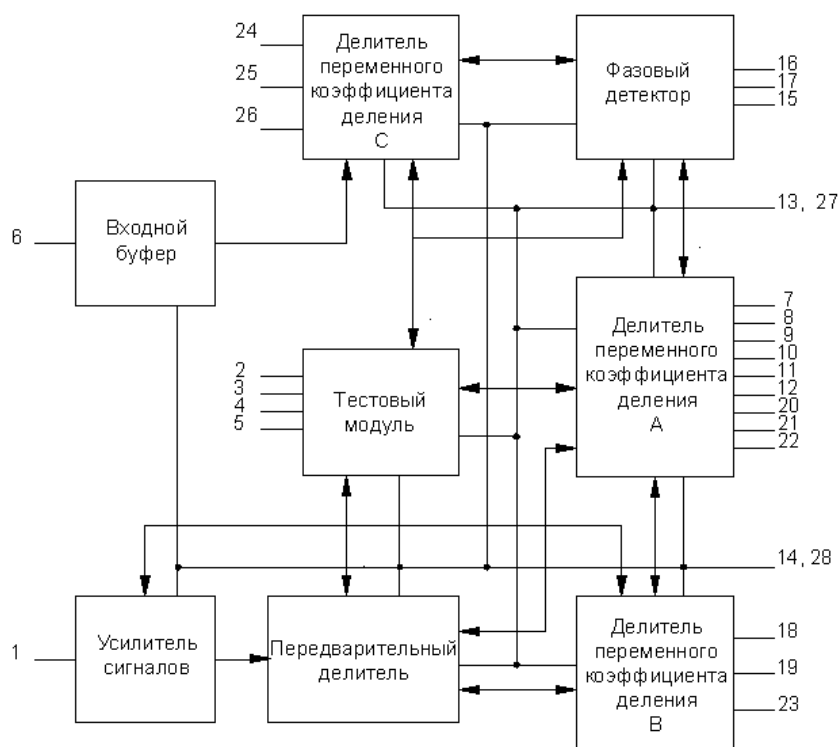
Рисунок 1. Структурная схема синтезатора частоты 1508ПЛ7У
