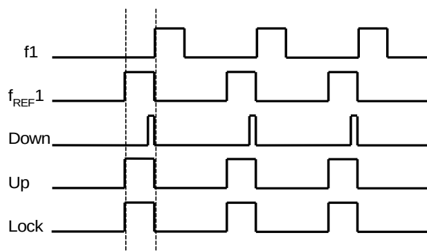
Рисунок 3. Сигналы ведомого генератора опережают сигналы опорного генератора
