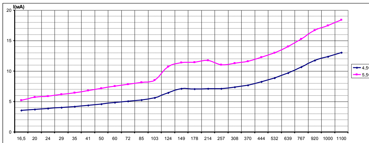
Рис. 6. Типовая зависимость тока потребления от входной частоты при напряжении питания 4,5В и 5,5В
