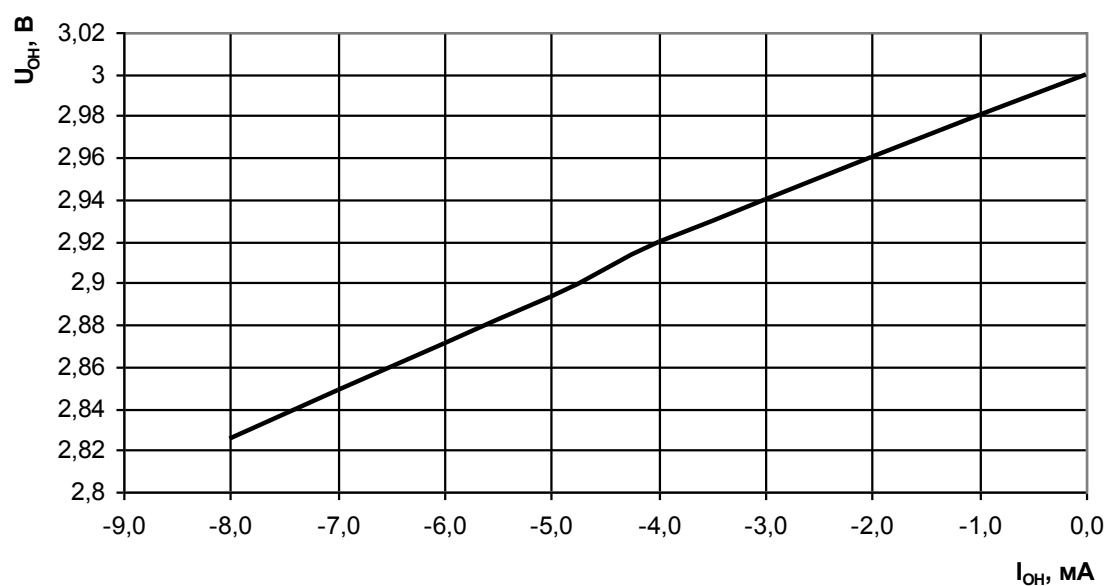
Рисунок 19 – Зависимость выходного напряжения высокого уровня от тока нагрузки при T = 25^\circ\text{C}
