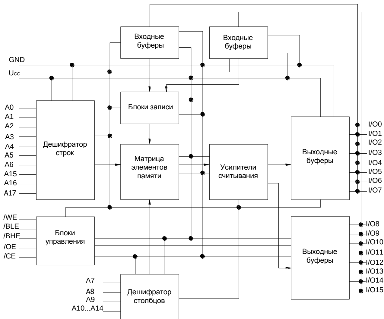
Рисунок 1 – Структурная блок-схема
