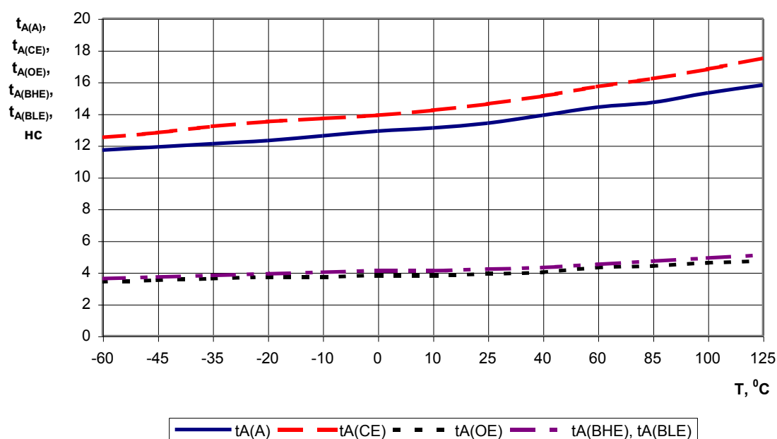
Рисунок 27 – Зависимость времени выборки адреса, t_{A(A)} , времени выборки по сигналу /CE, t_{A(CE)} , времени выборки по сигналу /OE, t_{A(OE)} , времени выборки по сигналу /BLE, t_{A(BLE)} , времени выборки по сигналу /BHE, t_{A(BHE)} , от температуры при U_{CC} = 3,0 В
