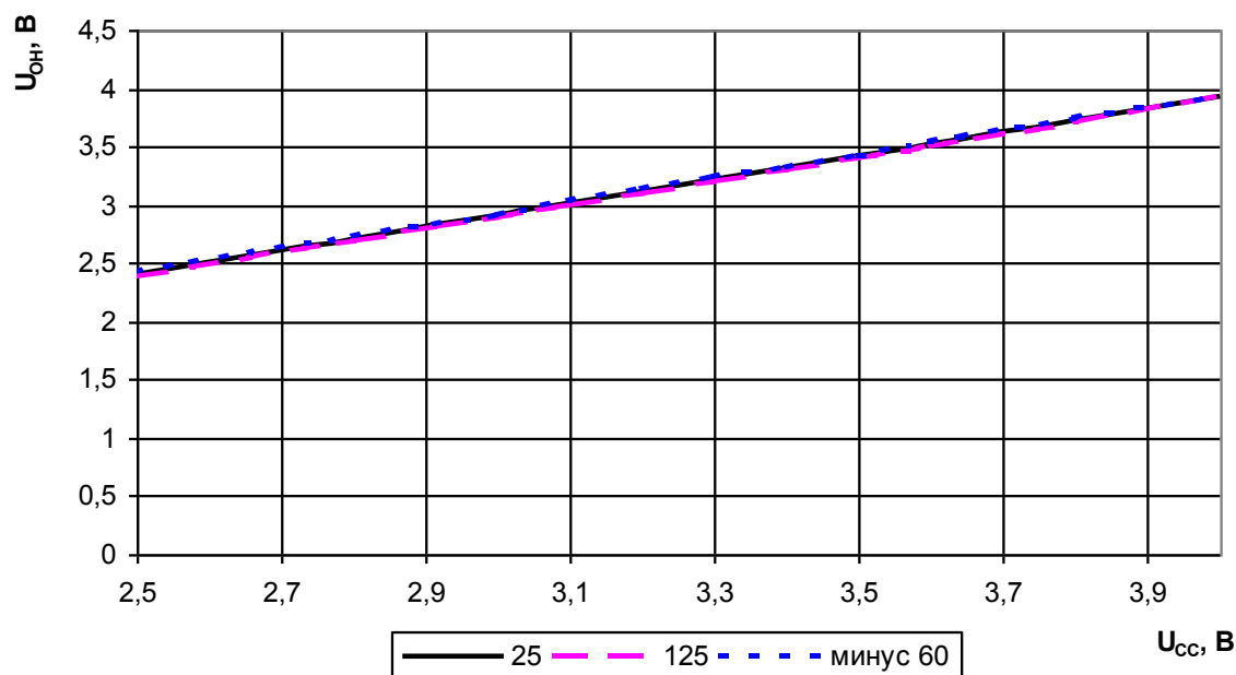
Рисунок 17 – Зависимость выходного напряжения высокого уровня от напряжения питания, при: I_{OH} = \text{минус } 4 мА
