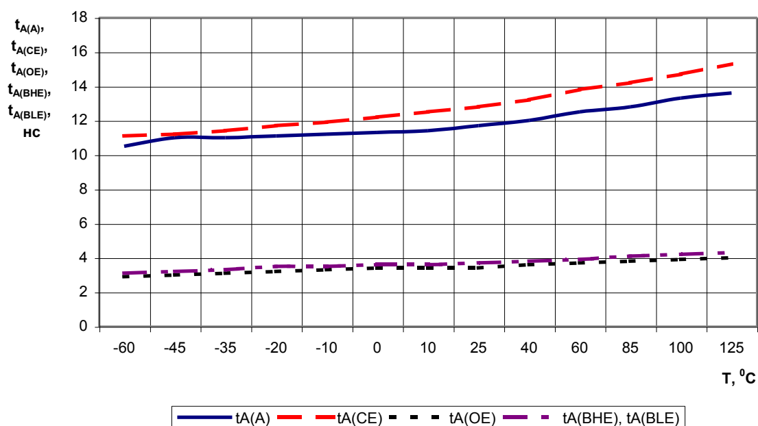
Рисунок 26 – Зависимость времени выборки адреса, t_{A(A)} , времени выборки по сигналу /CE, t_{A(CE)} , времени выборки по сигналу /OE, t_{A(OE)} , времени выборки по сигналу /BLE, t_{A(BLE)} , времени выборки по сигналу /BHE, t_{A(BHE)} , от температуры при U_{CC} = 3,6 В
