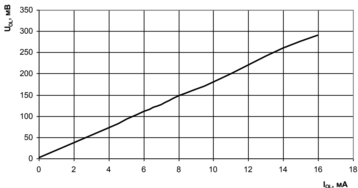
Рисунок 18 – Зависимость выходного напряжения низкого уровня от тока нагрузки при T = 25^\circ\text{C}
