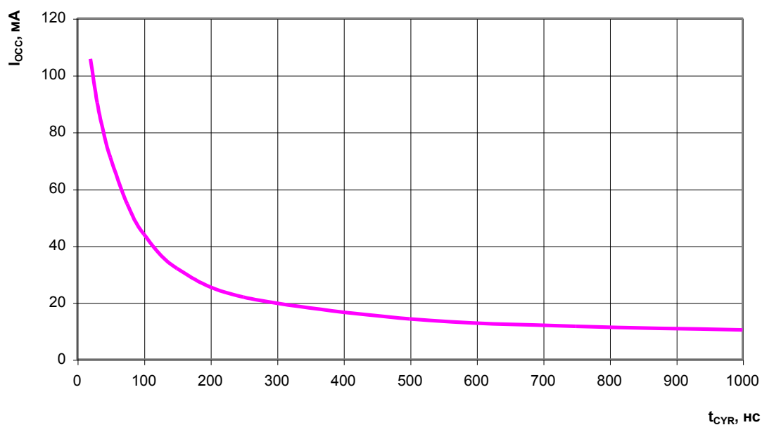
Рисунок 21 – Зависимость динамического тока потребления от времени цикла считывания информации t_{CYR} при U_{CC} = 3,6 В, T = 25 °C
