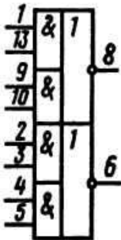
Условное графическое обозначение К530ЛР11
