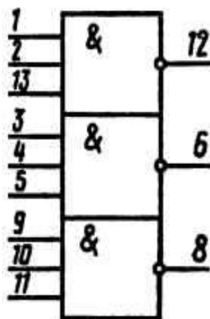
Условное графическое обозначение К530ЛИЗ
