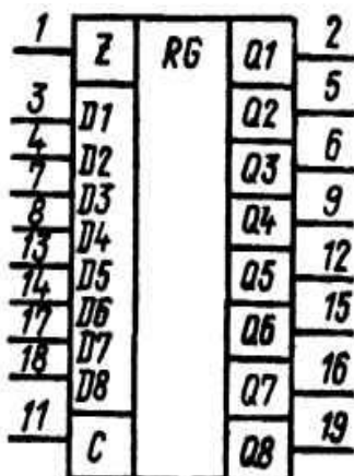
Условное графическое обозначение К530ИР22
