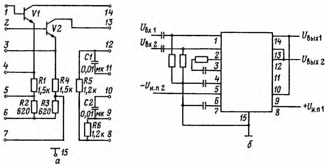
Принципиальная схема ИМС 265УВ4, К265УВ4 (а) и пример ее использования в балансном усилителе (б)
