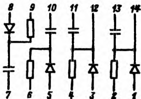
Электрическая схема К204НК1
