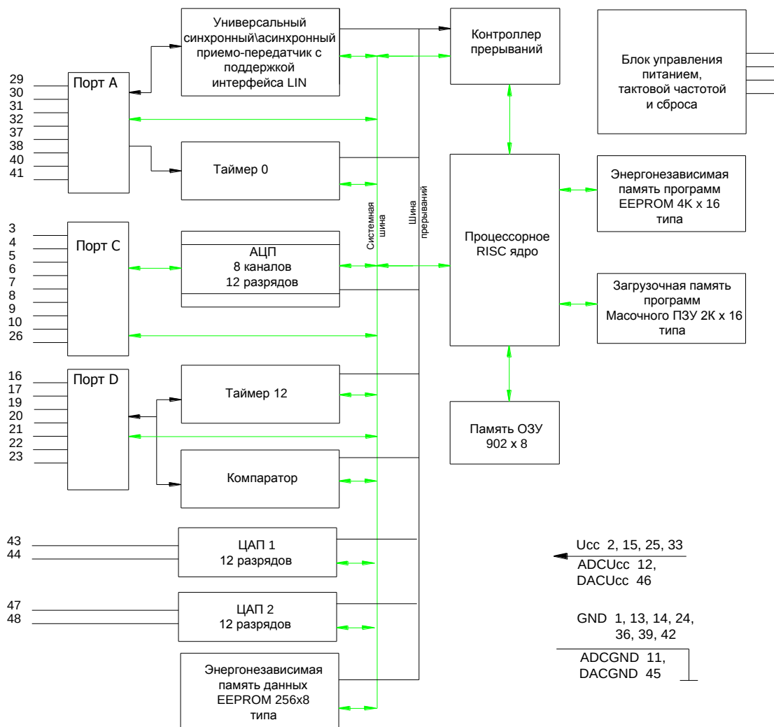
Рисунок 3 – Структурная блок-схема. Номера выводов указаны для микросхемы 1886BE6(61)У. Номера выводов для микросхемы 1886BE6(61)У1 см. в таблице
