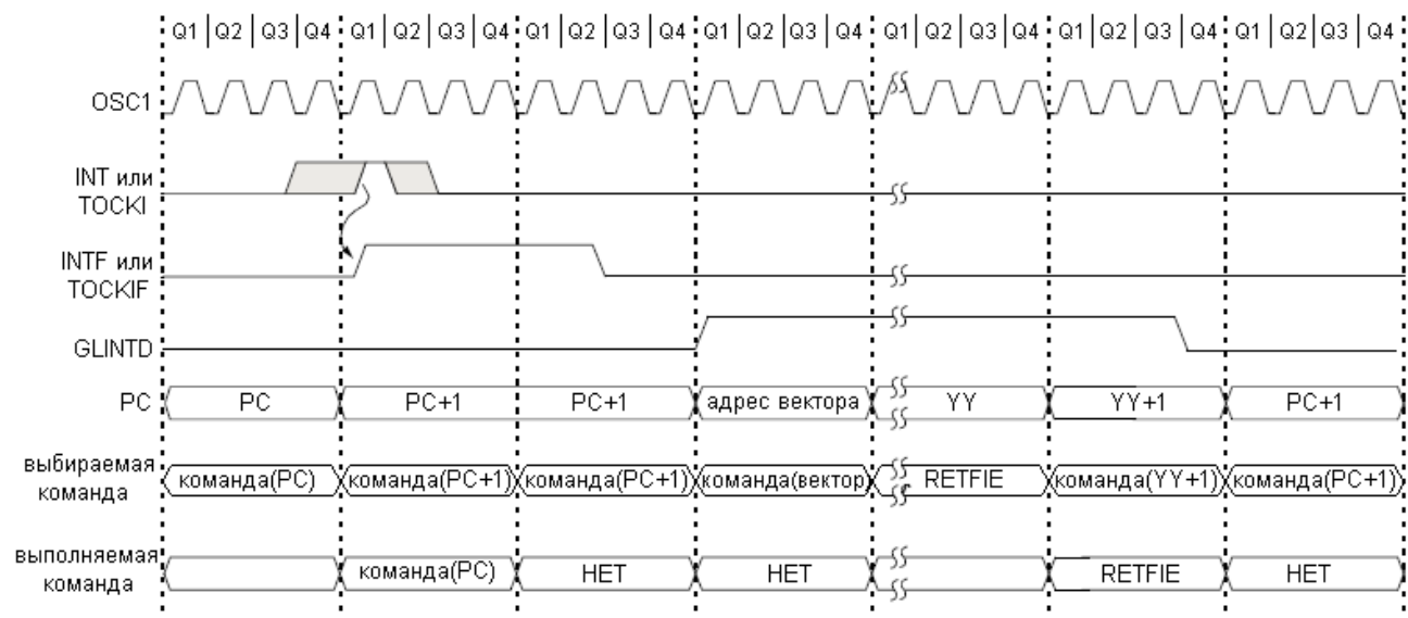
Рисунок 15 – Временная диаграмма обработки прерываний от выводов INT или T0CLK
