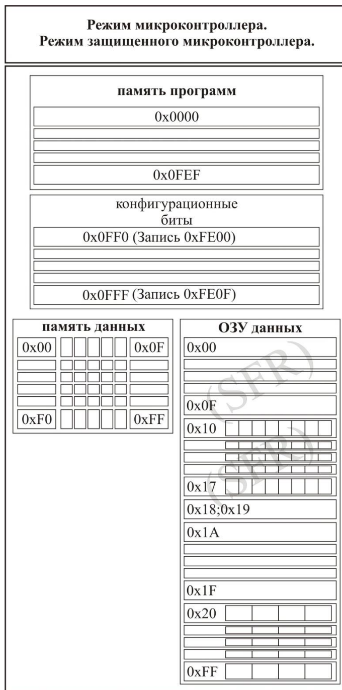
Рисунок 17 – Распределение памяти в различных режимах
