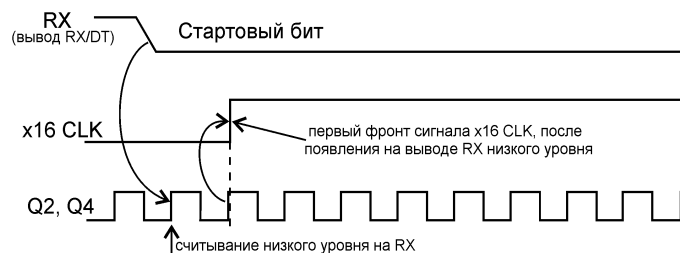
Рисунок 38 – Обнаружение стартового бита
