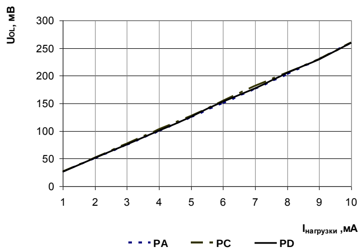
Рисунок 65 – Зависимость выходного напряжения низкого уровня на выводах PA, PC, PD, от тока нагрузки, при: T = 25^{\circ}\text{C} , U_{CC} = 4,5 \text{ В}
