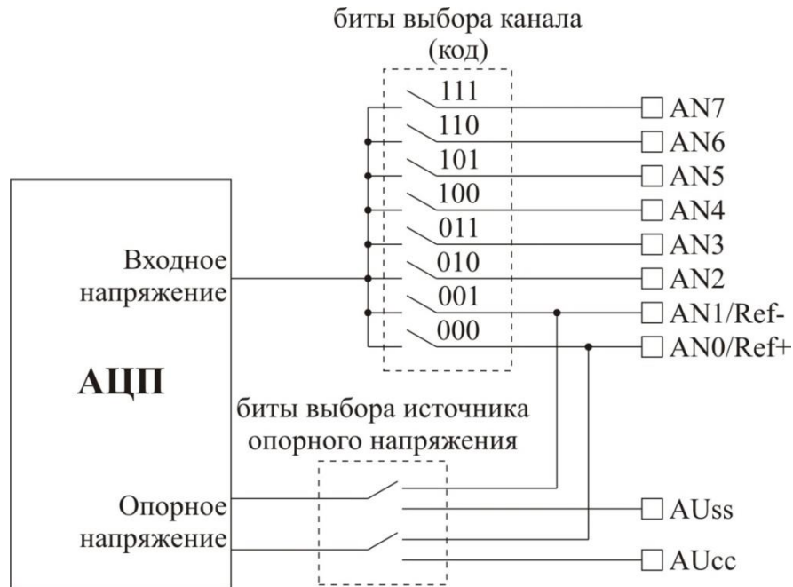
Рисунок 42 – Блок-схема модуля АЦП
