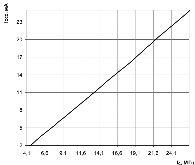
Рисунок 58 – Зависимость динамического тока потребления от частоты следования синхроимпульсов ( f_c ), при: T = 25^\circ\text{C} , U_{CC} = 5,5 \text{ В}
