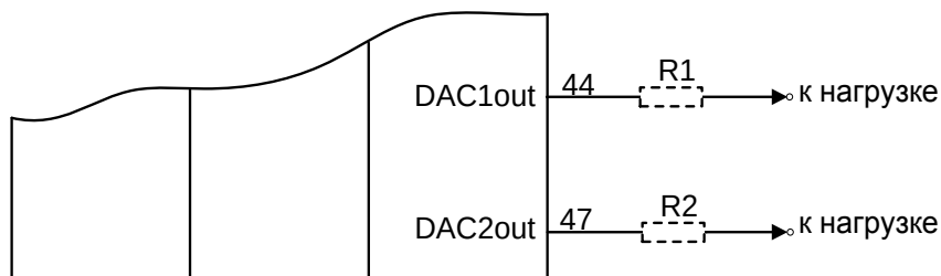
Рисунок 47 – Типовая схема включения микроконтроллера при использовании блока ЦАП
