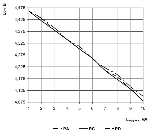
Рисунок 64 – Зависимость выходного напряжения высокого уровня на выводах PA, PC, PD, от тока нагрузки, при: T = 25^\circ\text{C} , U_{CC} = 4,5 В
