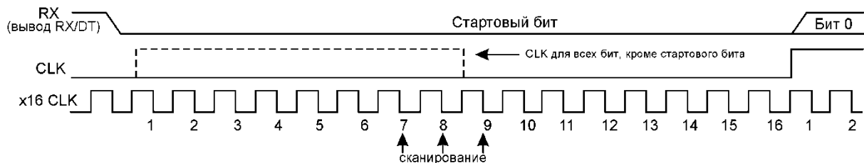
Рисунок 37 – Схема сканирования вывода PAx/RXx/DTx
