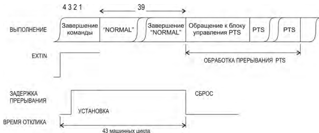
Рисунок 6.4 – Время реагирования на прерывание PTS
