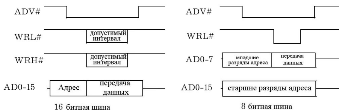
Рисунок 13.18 – Временные соотношения для режима Address Valid with Write Strobe
