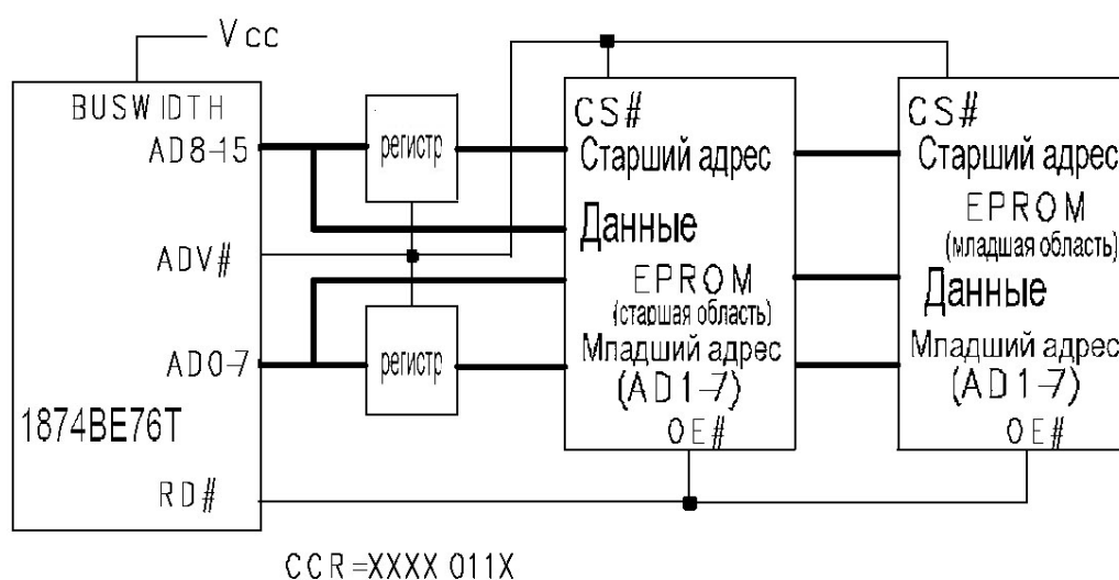
Рисунок 13.17 – 16 битная система с EPROM
