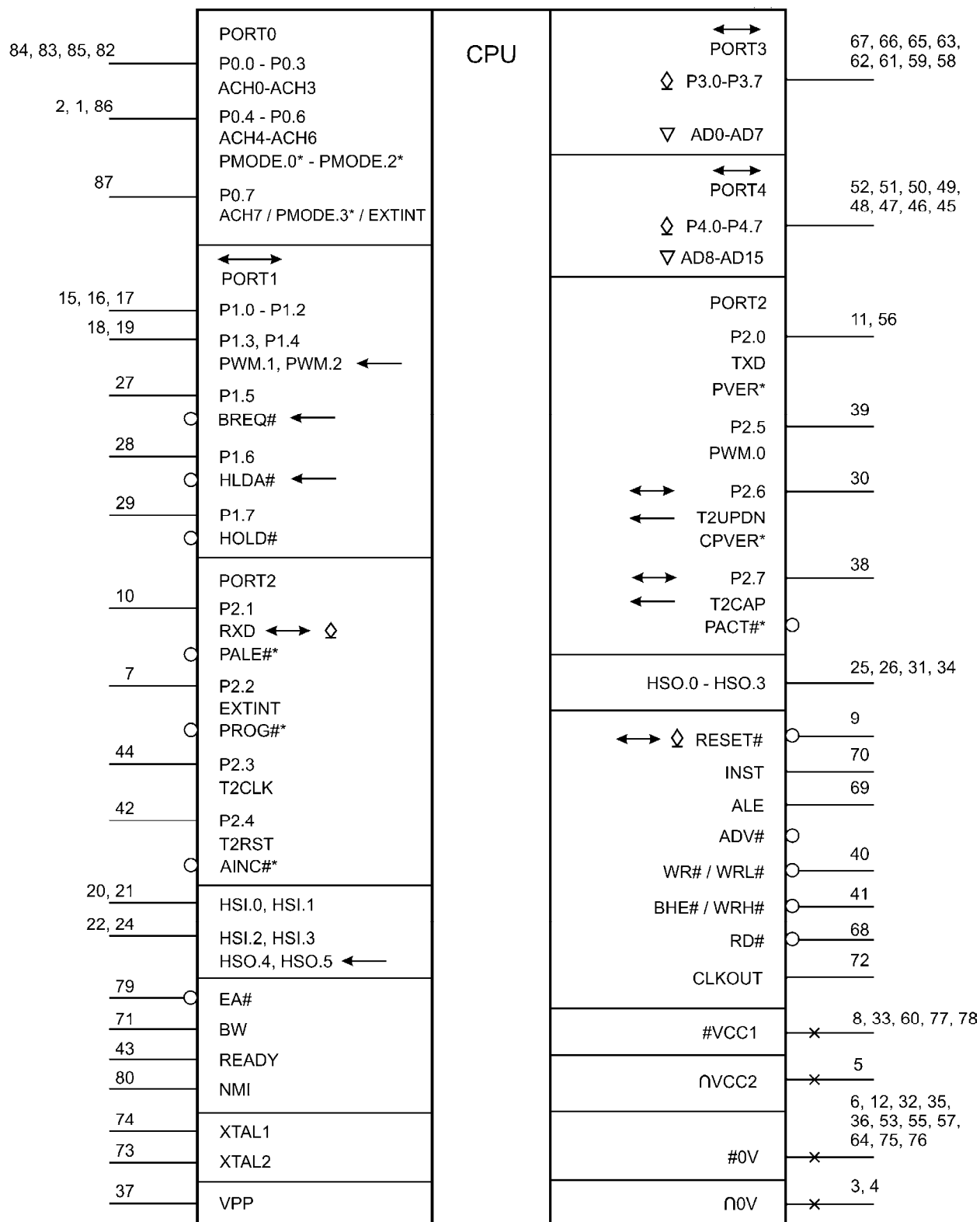
Рисунок 2.3 – Условное графическое изображение микросхем 1874BE76T, 1874BE06T
