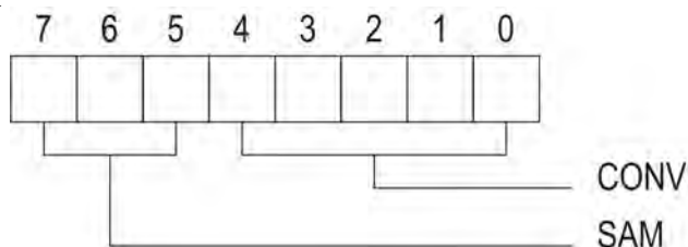
Рисунок 10.2 - Регистр AD_TIME
