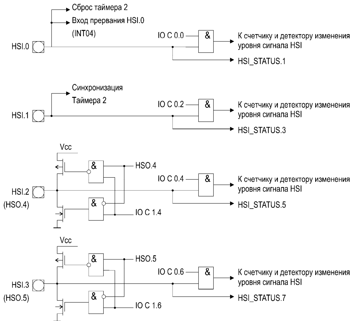
Рисунок 9.7 – Возможные входы HSI
