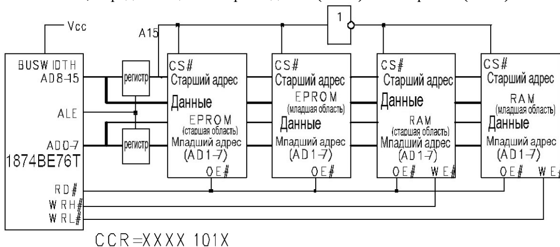
Рисунок 13.13 – Пример 16-битной системы с однокбайтной записью в RAM
