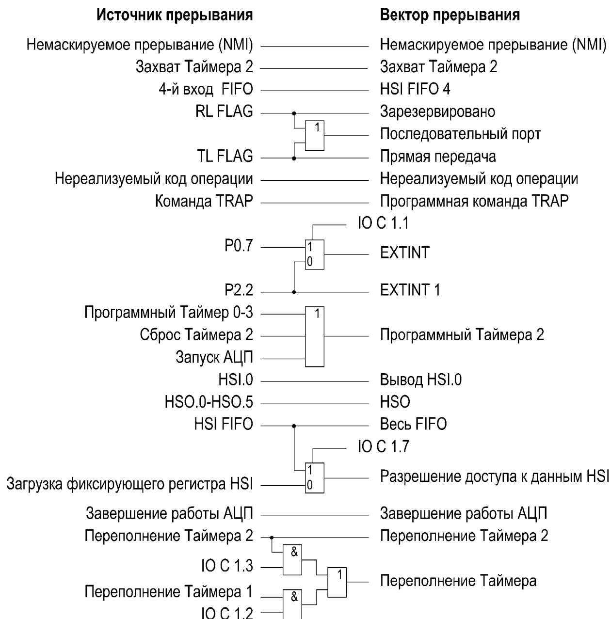
Рисунок 6.5 – Источники прерываний
