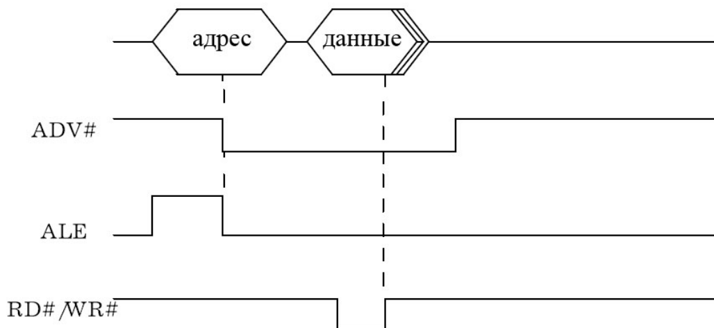
Рисунок 13.15 – Сравнение шинных циклов ALE и ADV#
