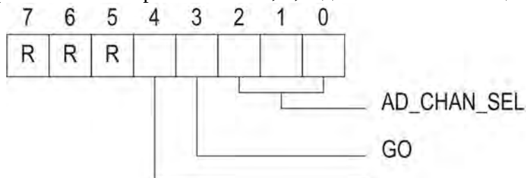
Рисунок 10.4 – Регистр AD_COMMAND
