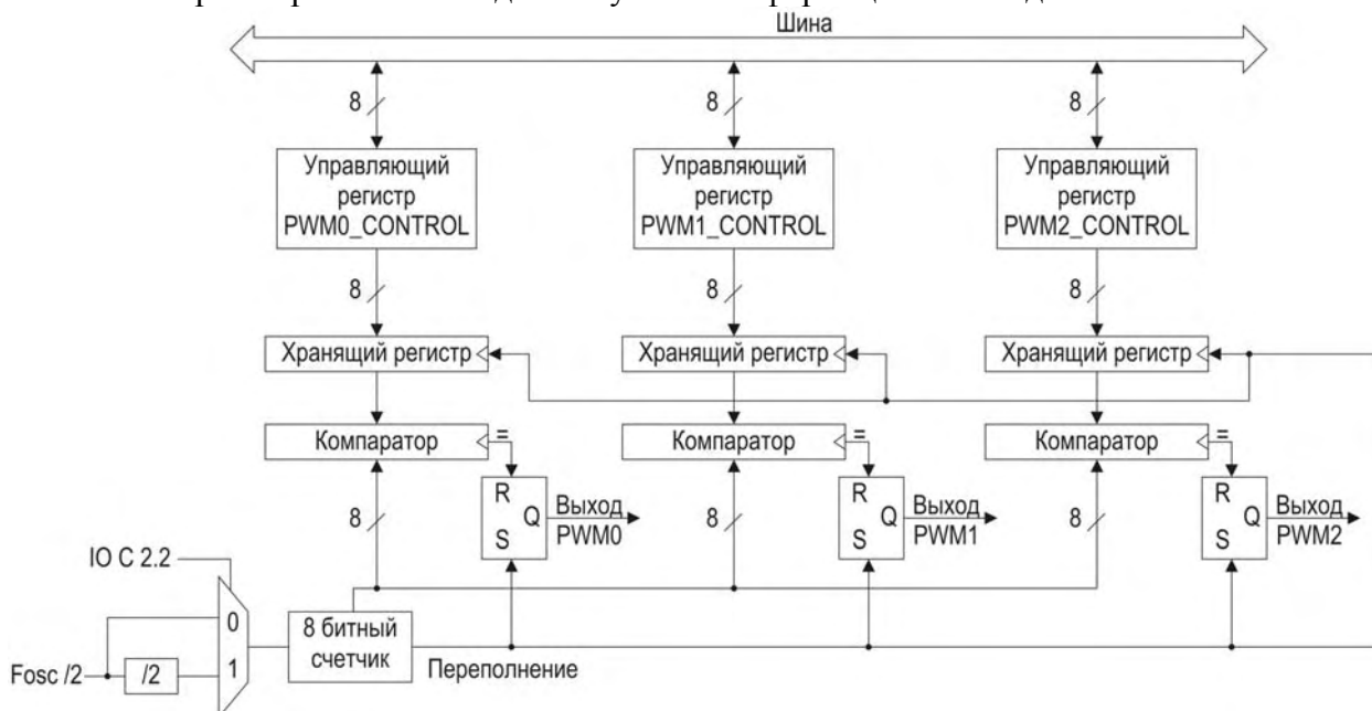
Рисунок 11.1 – Блок-схема модуля PWM
