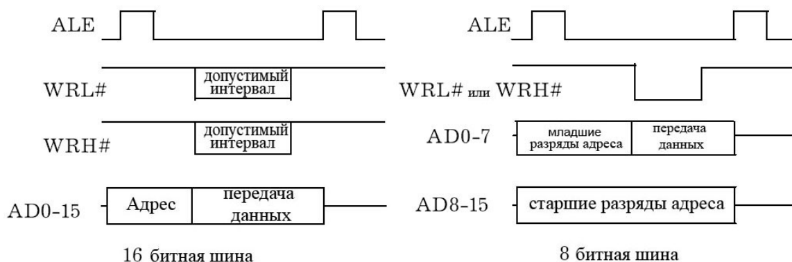
Рисунок 13.12 – Режим Write Strobe
