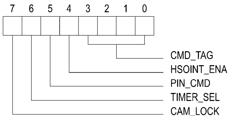
Рисунок 9.9 – Регистр HSO_COMMAND
