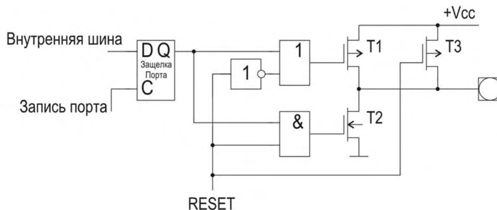
Рисунок 7.2 – Выходной вывод порта
