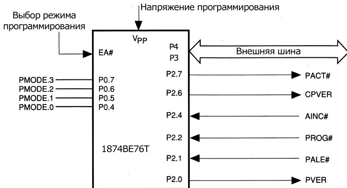
Рисунок 14.1 – Назначение выводов в режиме программирования
