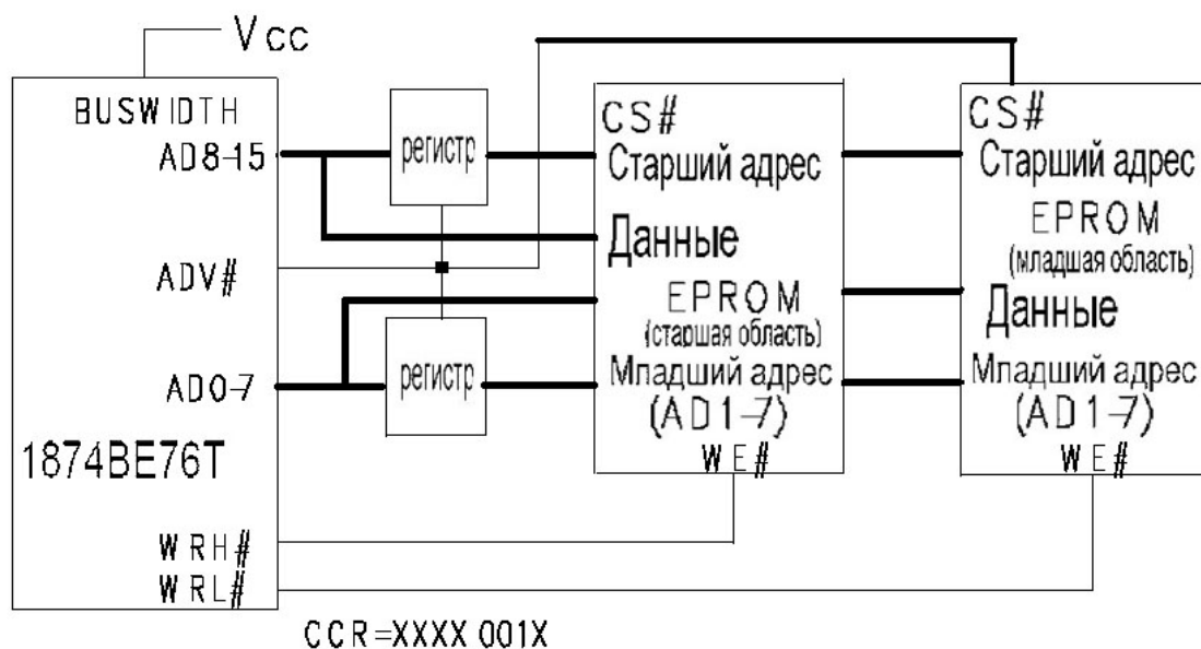
Рисунок 13.19 – 16-битная система с RAM
