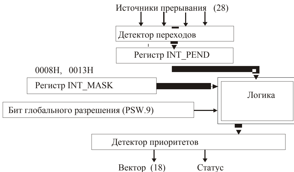
Рисунок 5.2 – Блок-схема системы прерываний
