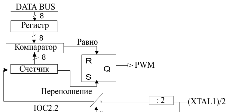
Рисунок 6-1 Выход с ШИМ
