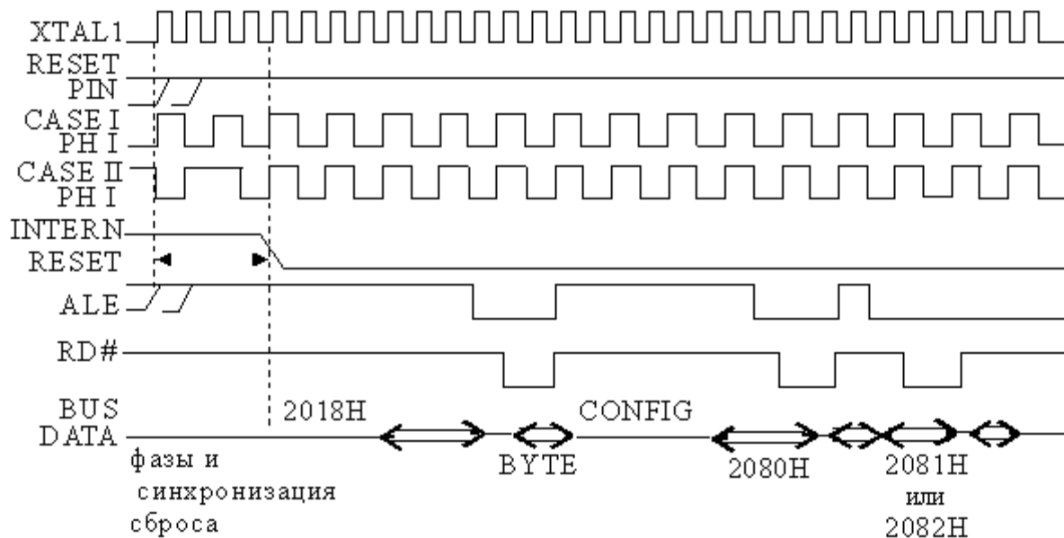
Рисунок 13.5 – Последовательность сброса
