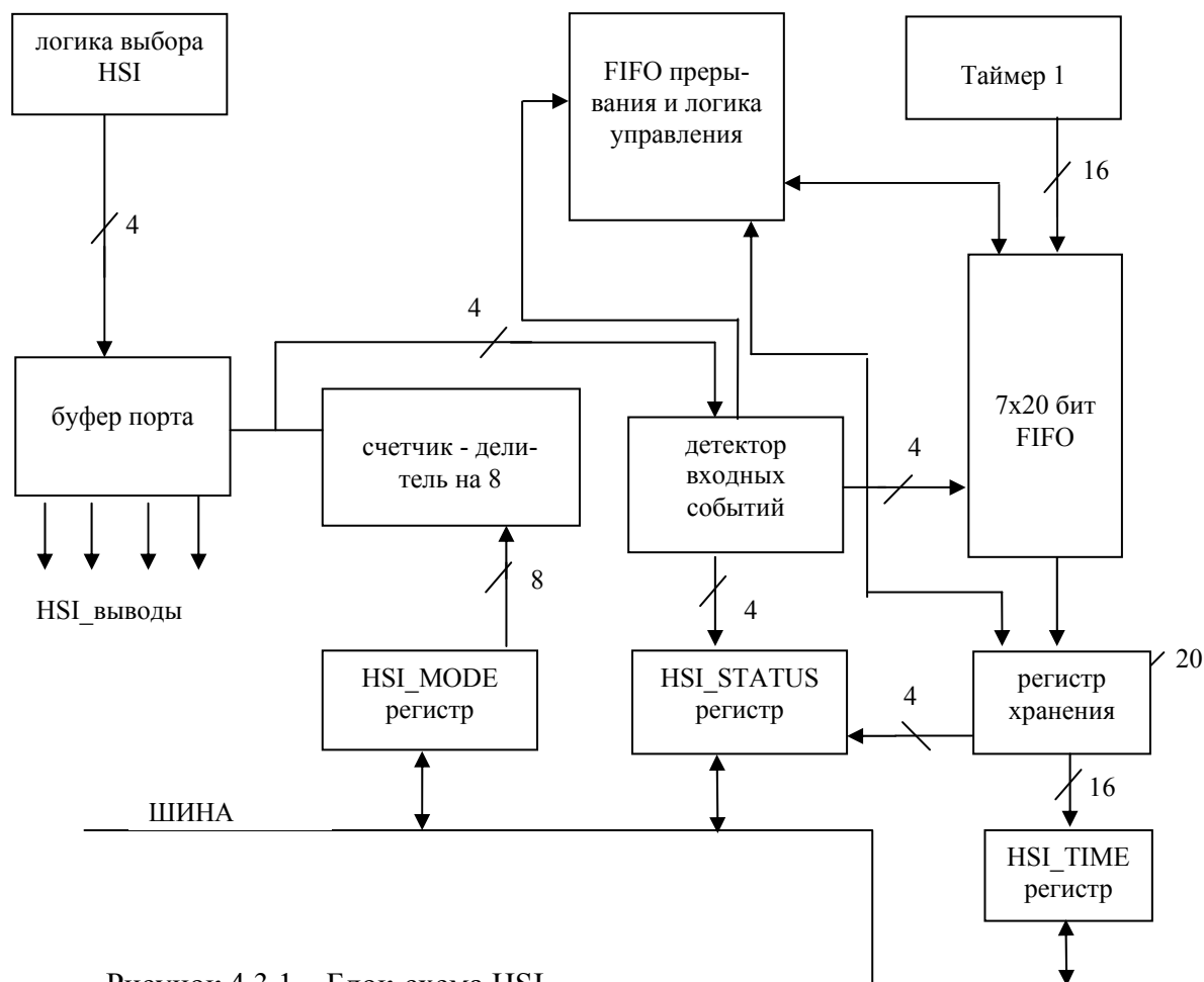
Рисунок 4.3.1 – Блок-схема HSI
