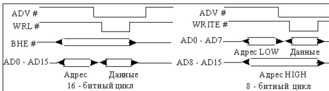
Рисунок 15.2.3 – Режим стробирования действительного адреса
