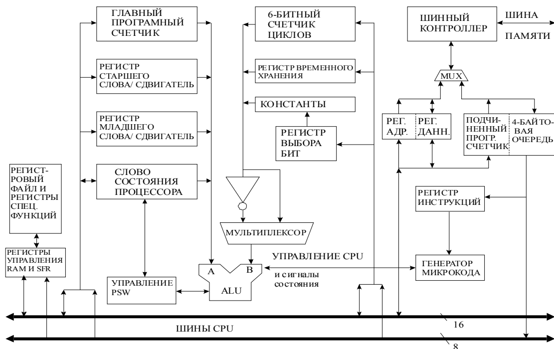
Рисунок 2.4.1 – Блок-схема РАЛУ
