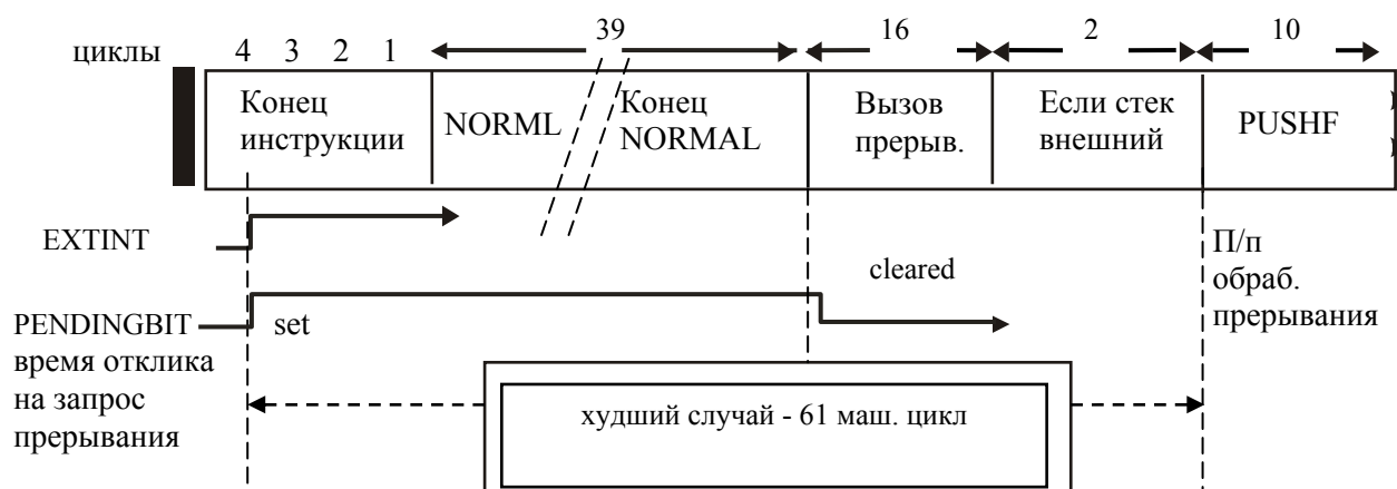
Рисунок 5.4.1 - Время прерывания
