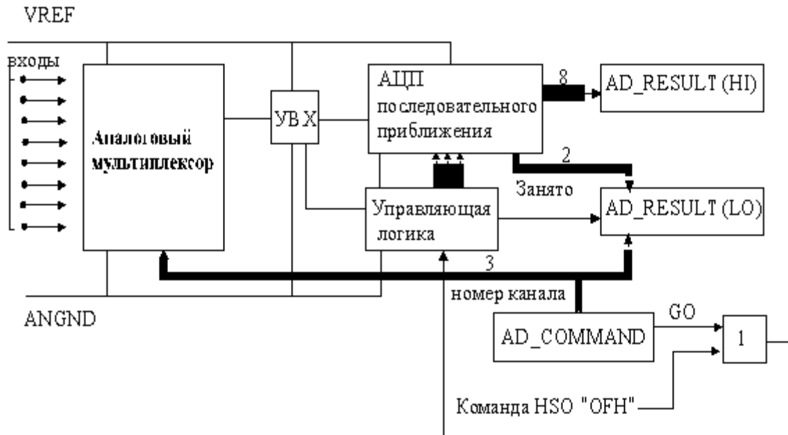
Рисунок 11.1 - Схема АЦП
