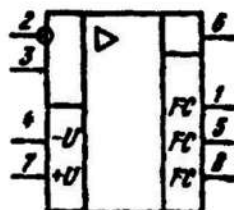
Условное графическое обозначение К153УД1А, К153УД101А
