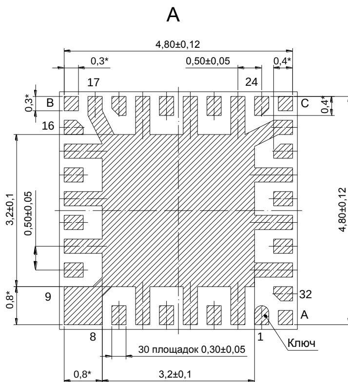
Рисунок 16 – Корпус 5102.32-2К
