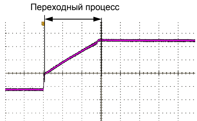
Рисунок 7 – Осциллограмма переходного процесса петли ФАПЧ с включенной функцией CSP. DN=0,1·INT
