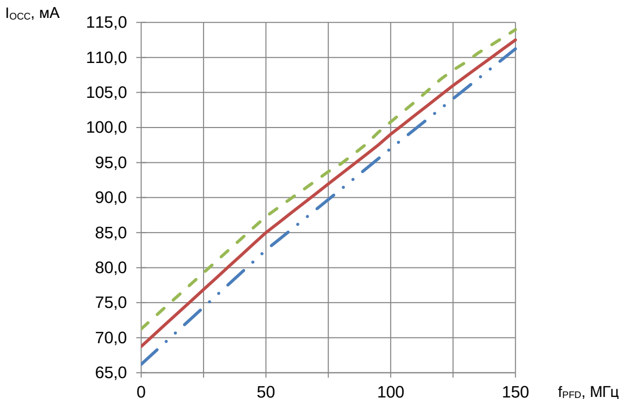
Рисунок 13 – Зависимость динамического тока потребления I_{OSS} от частоты сравнения фазового детектора f_{PFD} в целочисленном режиме, при U_{CC} = 3,3 В
