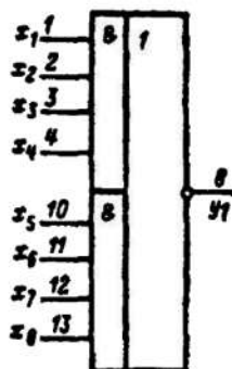
Условное графическое обозначение К136ЛР4
