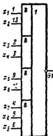
Условное графическое обозначение К136ЛРЗ
