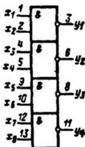
Условное графическое обозначение К136ЛАЗ
