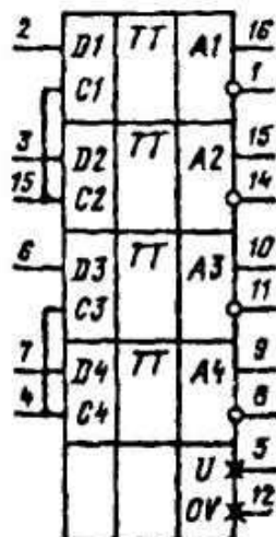
Условное графическое обозначение K133TM7
