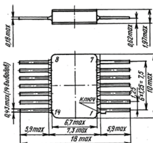
Корпус 401.14-5М
