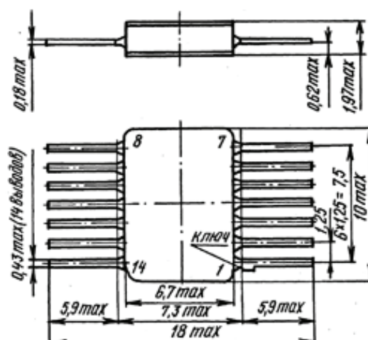
Корпус 401.14-5М
