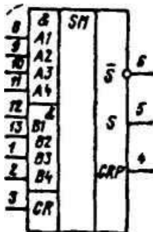
Условное графическое обозначение К13ЗИМ1
