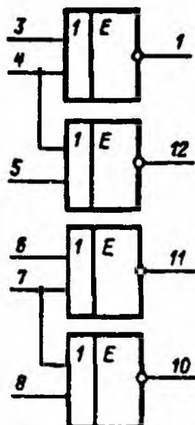
Условное графическое обозначение К114ЛД1
