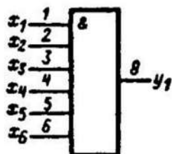
Условное графическое обозначение К109ЛИ1
