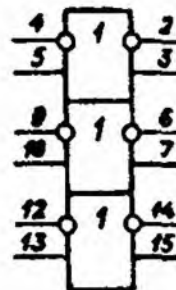
Условное графическое обозначение К100ЛП216
