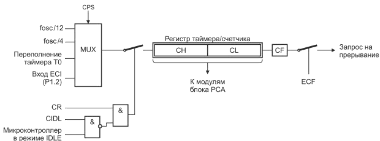
Рисунок 9.1 – Таймер/счетчик ТС блока PCA и источники его сигнала тактирования
