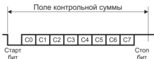
Рисунок 14.8 – Поле контрольной суммы
