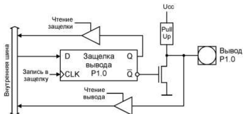
Рисунок 3.2 – Функциональная схема канала порта 1
