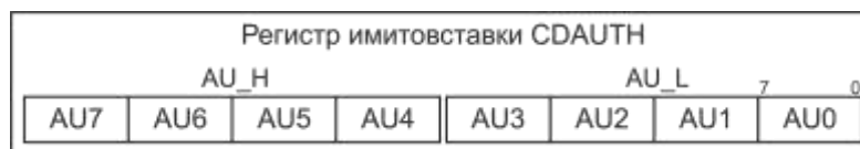
Рисунок 15.6 – Структура регистра CDAUTH
