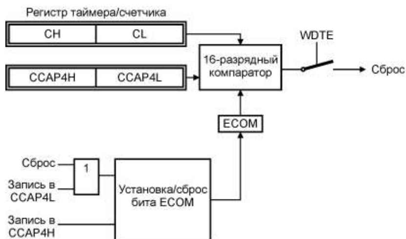
Рисунок 9.5 – Модуль 4 блока PCA в режиме сторожевого таймера
