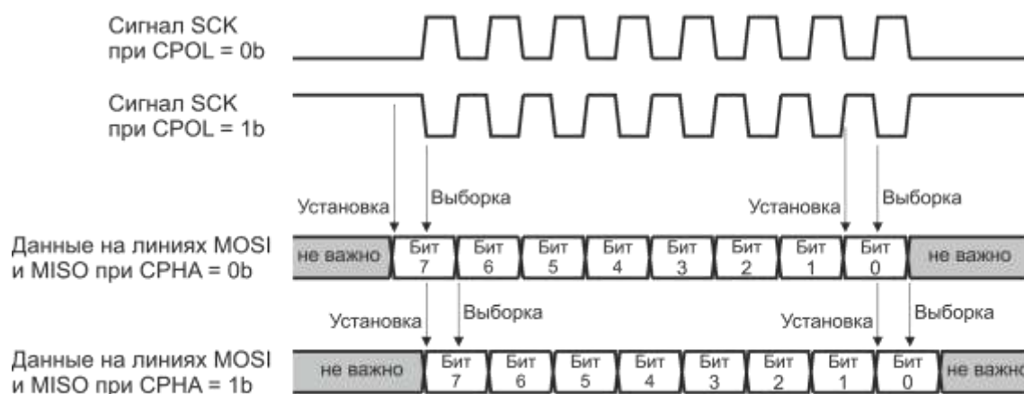
Рисунок 12.3 – Временные диаграммы передач данных в разных режимах
