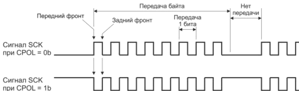
Рисунок 12.2 – Сигнал синхронизации SCK при разных состояниях бита CPOL
