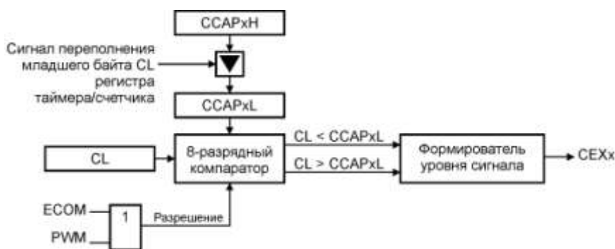
Рисунок 9.6 – Блок РСА в режиме широтно-импульсного модулятора
