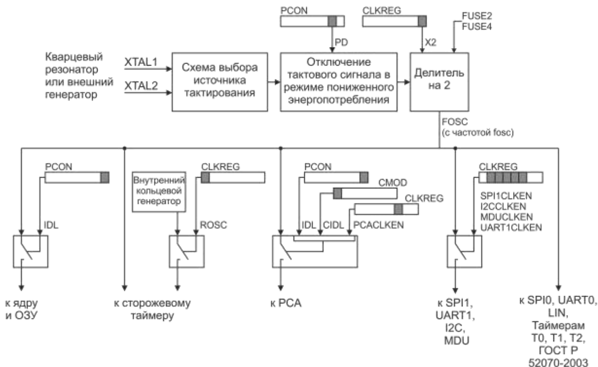
Рисунок 6.2 – Схема тактирования микроконтроллера
