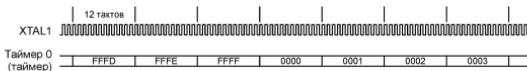
Рисунок 8.1 – Работа таймера/счетчика T0 в режиме таймера
