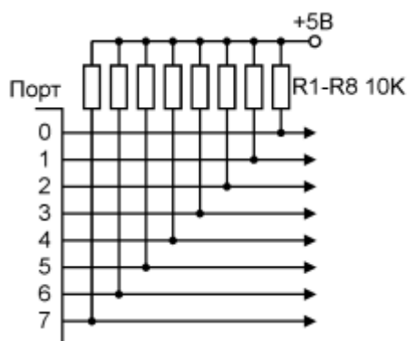
Рисунок 3.6 – Использование линий порта для ввода/вывода
