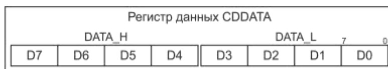
Рисунок 15.1 – Структура регистра CDDATA
