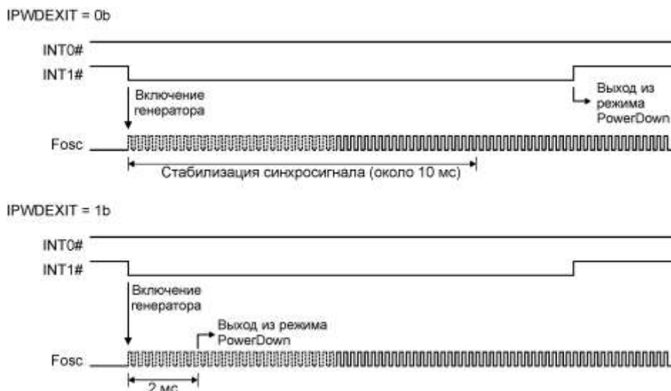
Рисунок 19.1 – Выход из режима PowerDown
