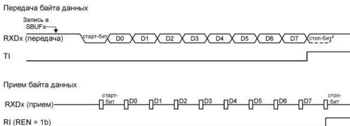
Рисунок 11.2 – Временная диаграмма передачи байта в режиме 1
