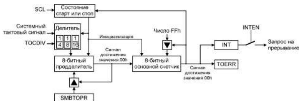
Рисунок 13.14 – Функциональная схема счетчика времени ожидания
