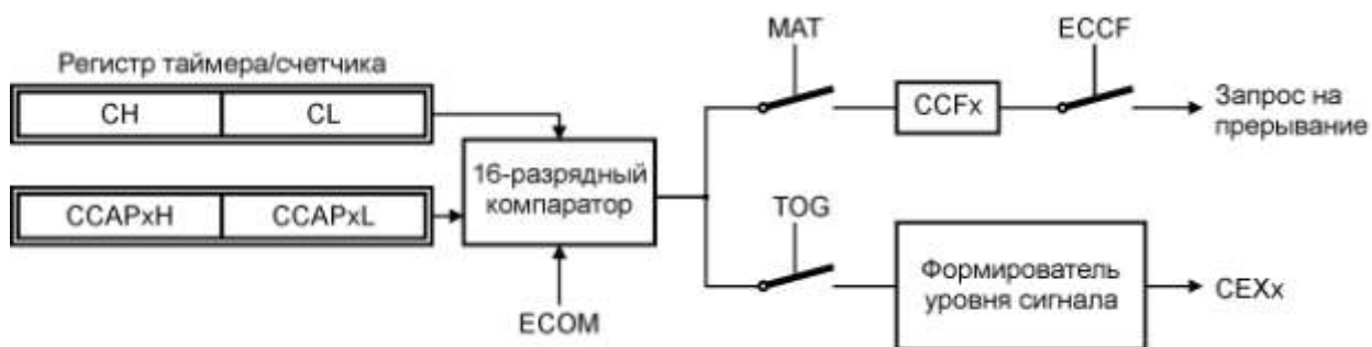
Рисунок 9.4 – Блок PCA в режиме скоростного вывода
