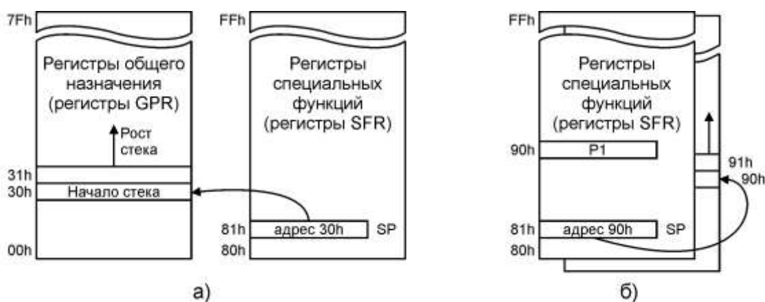
Рисунок 4.3 – Адресация указателем стека SP
