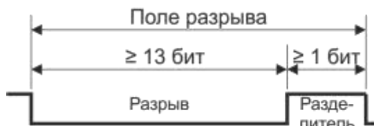
Рисунок 14.3 – Поле разрыва синхронизации
