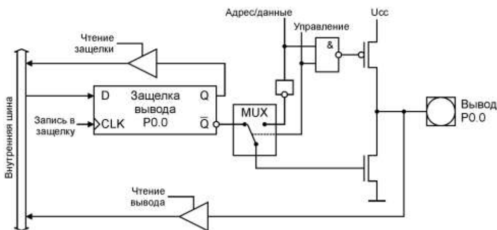
Рисунок 3.1 – Функциональная схема канала порта 0
