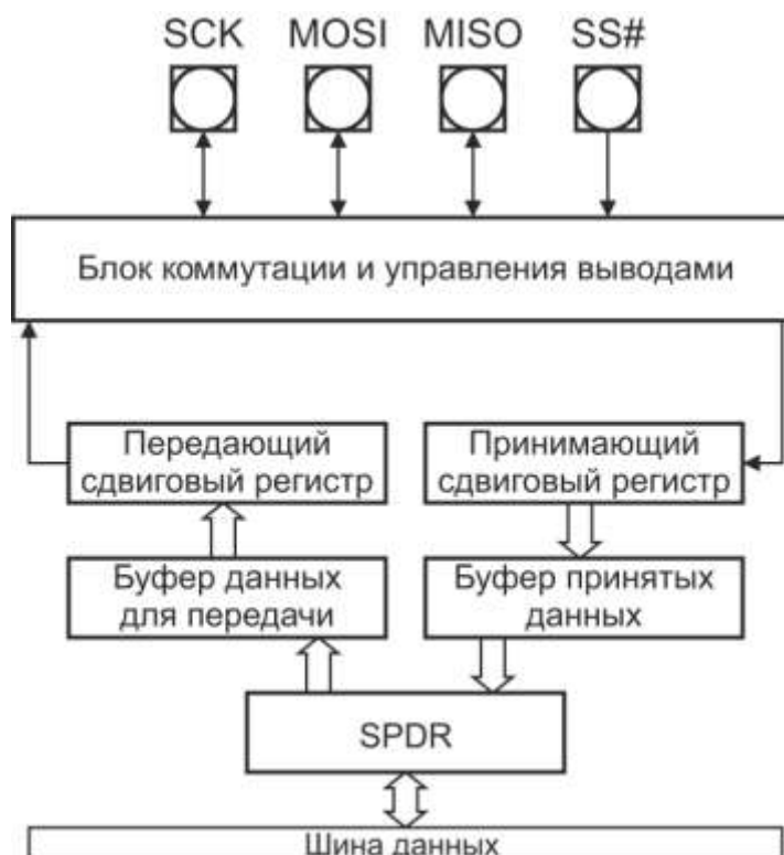
Рисунок 12.1 – Структурная схема взаимодействия блоков модуля SPI
