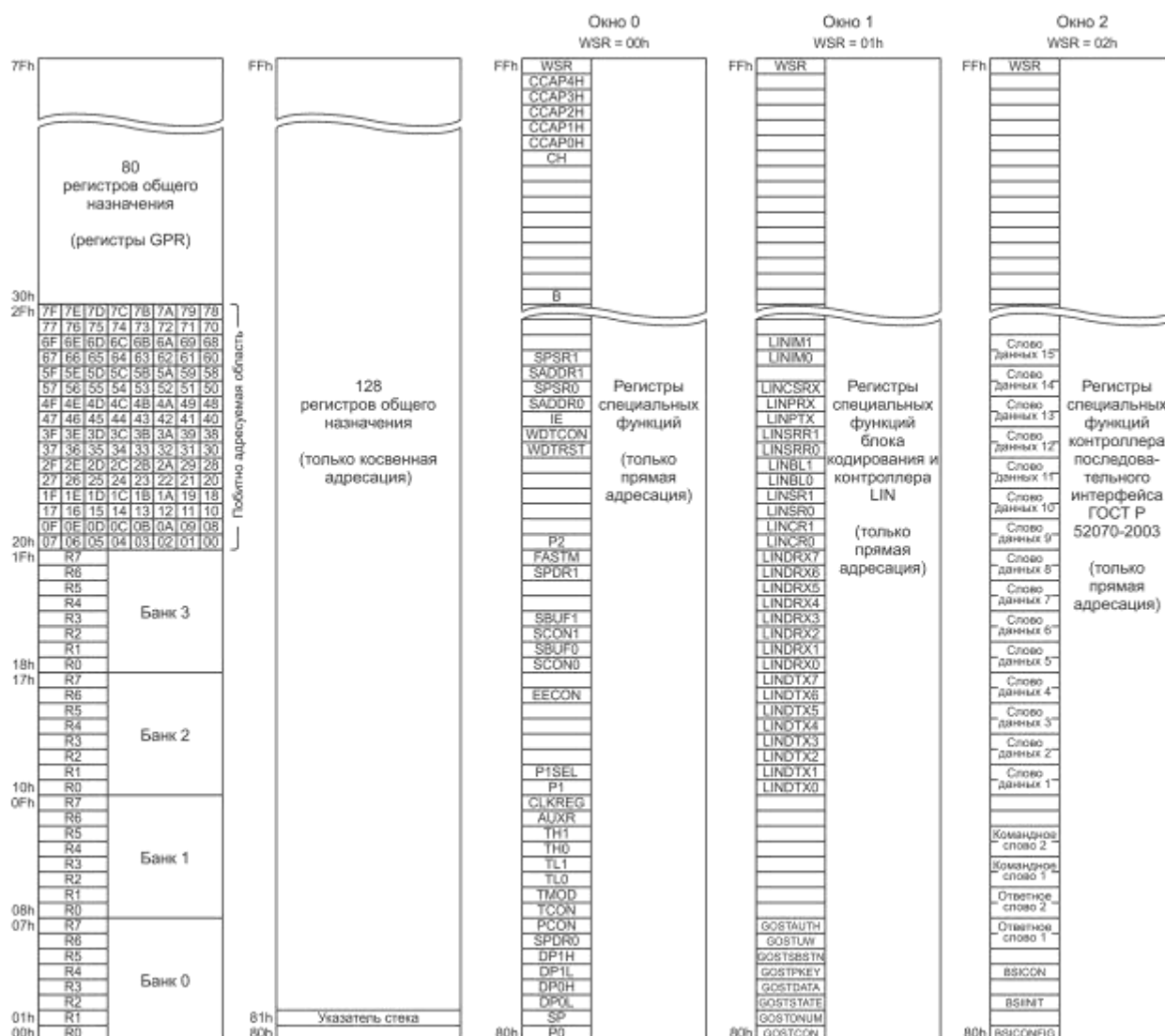
Рисунок 4.1 – Оконная организация ОЗУ
