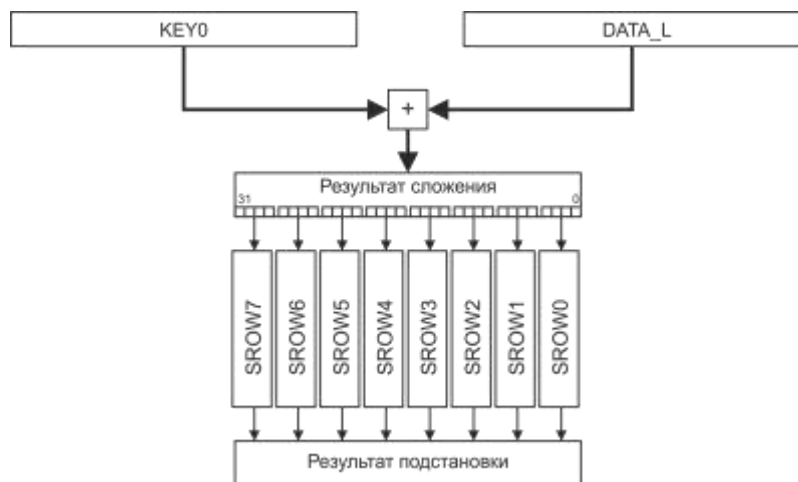
Рисунок 15.4 – Частичная функциональная схема алгоритма режима простой замены
