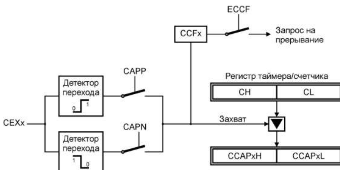
Рисунок 9.2 – Схема функционирования модуль x для режимов захвата
