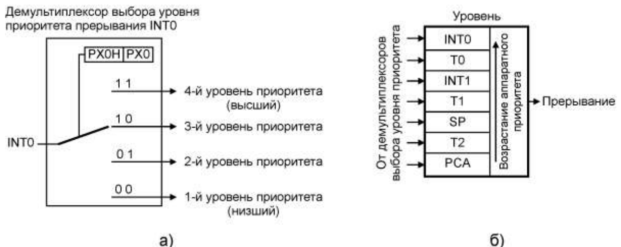
Рисунок 17.1 – Механизмы ранжирования векторов прерываний
