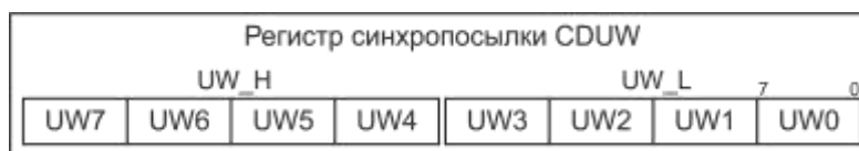
Рисунок 15.5 – Структура регистра CDUW
