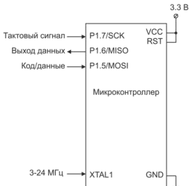
Рисунок 20.2 – Схема включения при последовательном программировании
