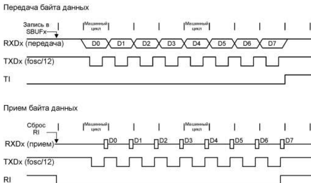
Рисунок 11.1 – Временная диаграмма передачи байта в режиме 0
