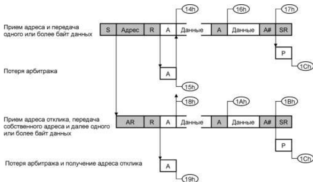
Рисунок 13.22 – Режим FS ведомого передатчика
