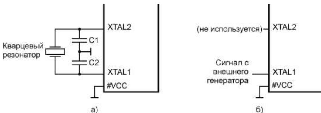
Рисунок 6.1 – Схемы подключения источника
