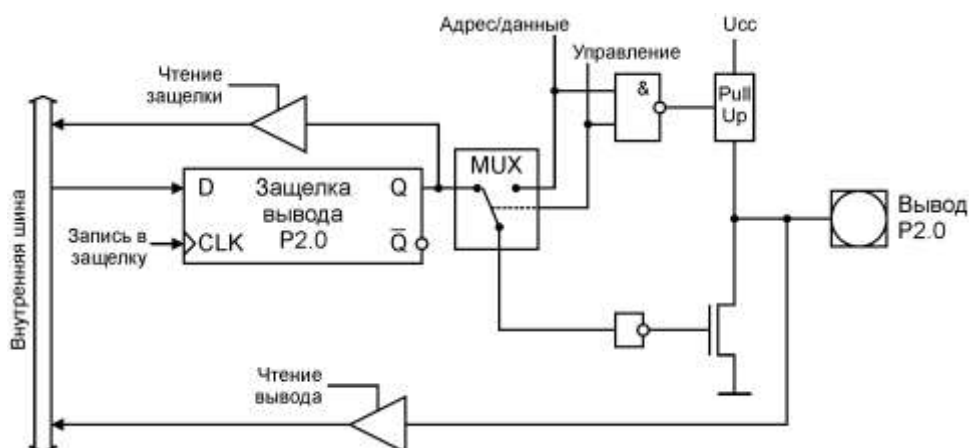
Рисунок 3.3 – Функциональная схема канала порта 2
