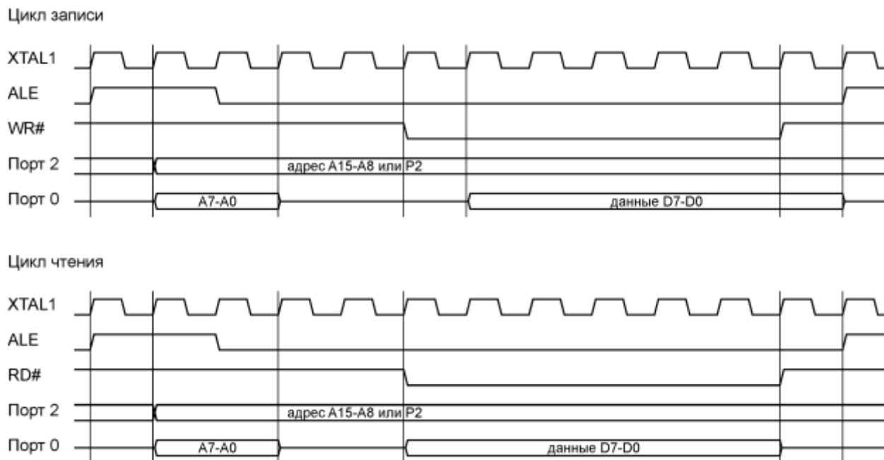
Рисунок 5.3 – Обращение к внешней памяти программ. Циклы чтения и записи
