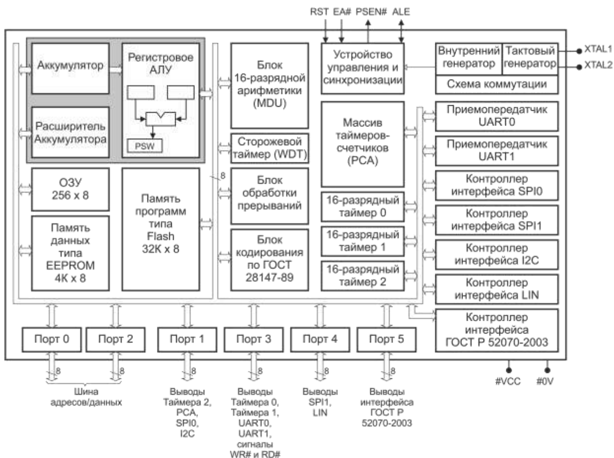
Рисунок 2.1 – Структурная схема 1882BM1T
