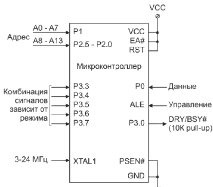
Рисунок 20.1 – Схема включения при параллельном программировании
