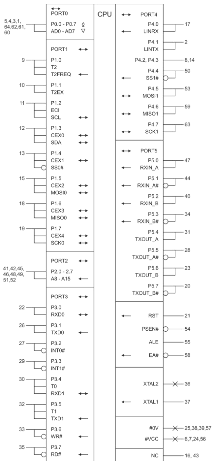
Рисунок 1.1 – Условное графическое обозначение ИС в корпусе 4203.64-1
