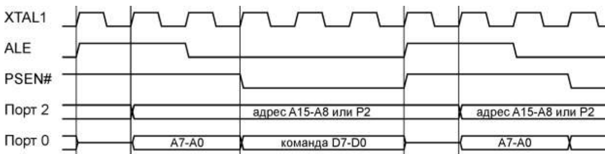
Рисунок 5.2 – Обращение к внешней памяти программ. Цикл чтения
