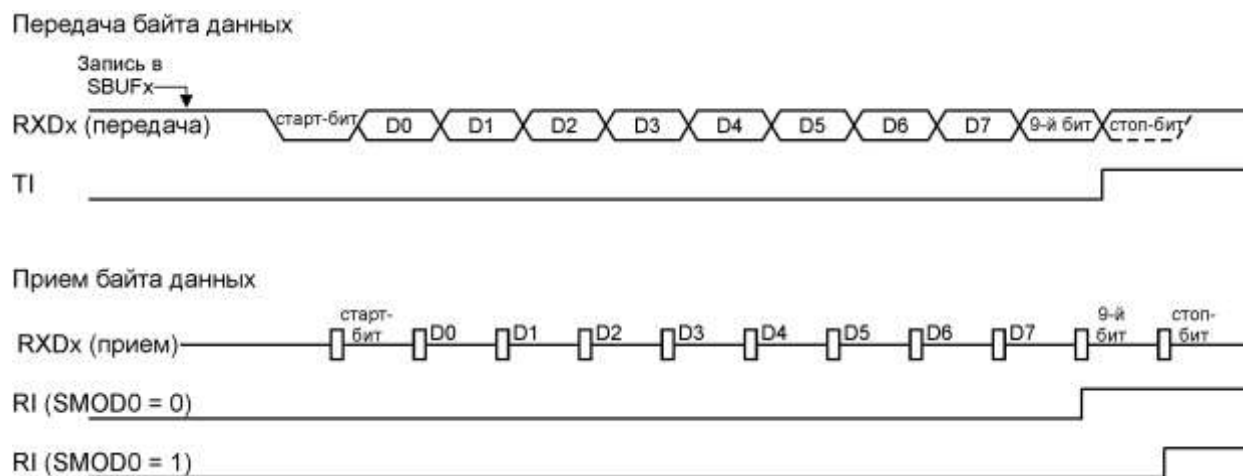
Рисунок 11.3 – Временная диаграмма передачи байта в режиме 2
