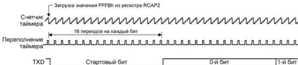
Рисунок 8.3 – Тактирование передачи
