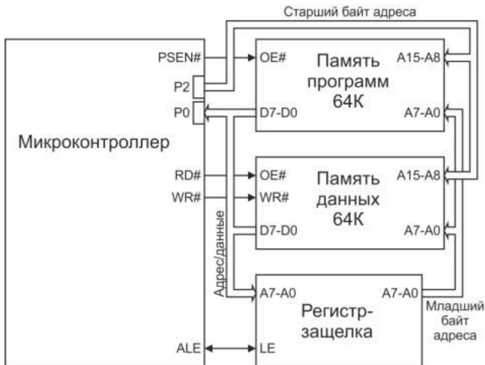
Рисунок 5.1 – Подключение внешней памяти
