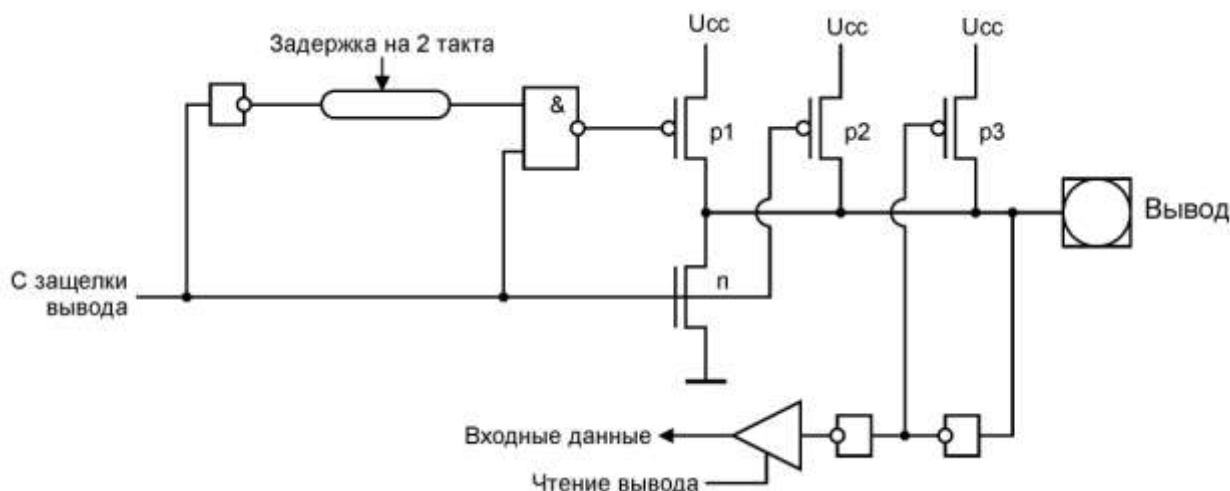
Рисунок 3.5 – Подтягивающая схема pull-up
