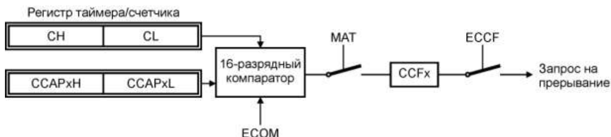
Рисунок 9.3 – Блок PCA в режиме 16-разрядного таймера
