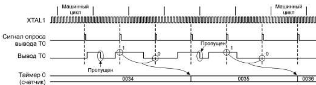
Рисунок 8.2 – Работа таймера/счетчика T0 в режиме счетчика
