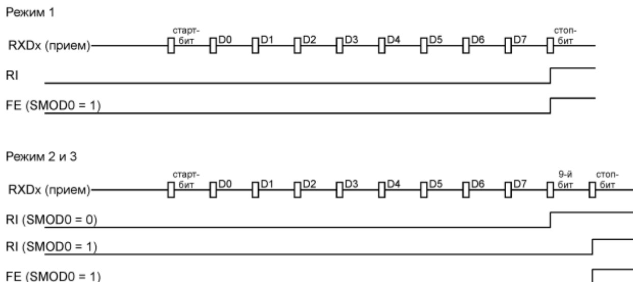
Рисунок 11.4 – Выставление флага FE при приеме некорректного стоп-бита
